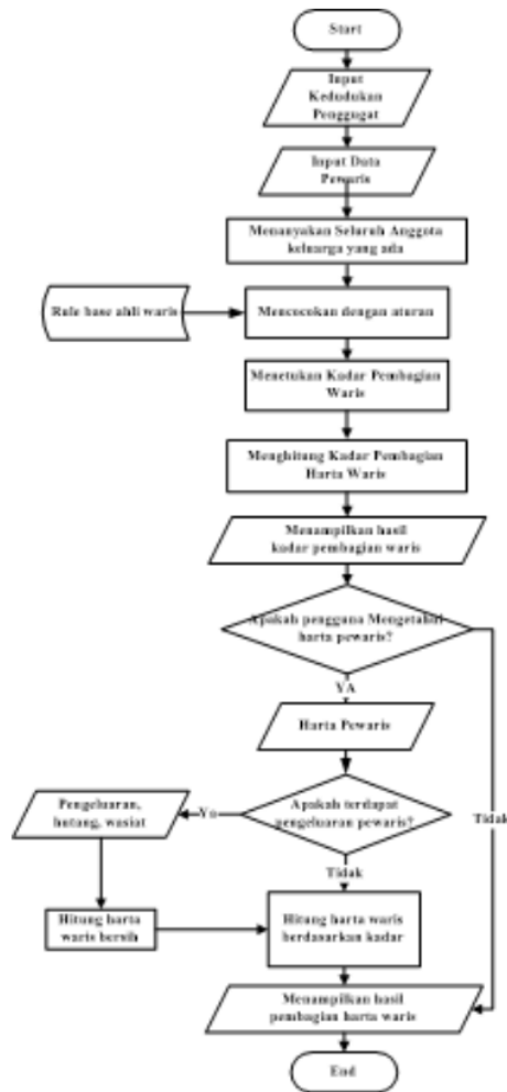
Gambar 1. Flowchart Sistem Pendukung Keputusan Pembagian Harta Waris
