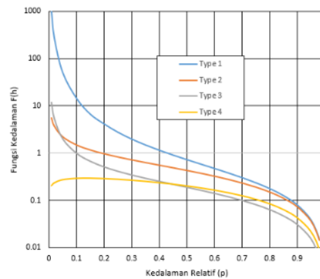
Gambar 2 Grafik hubungan kedalaman relatif (p) dan nilai F(h)
