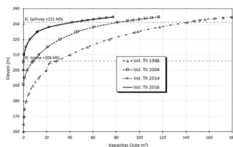
Gambar 3 Perkembangan Kurva H-V di Waduk Mrica 1988 – 2016
