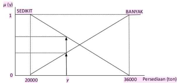
Gambar 6. Fungsi Keanggotaan Variabel Persediaan Semen PPC
