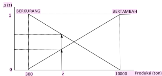
Gambar 7. Fungsi Keanggotaan Variabel Produksi Semen PPC
