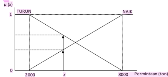
Gambar 5. Fungsi Keanggotaan Variabel Permintaan Semen PPC
