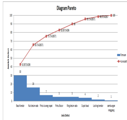
Gambar 3 Diagram Pareto Pada Water Test & Underframe (Sumber: Data Olahan, 2019)
