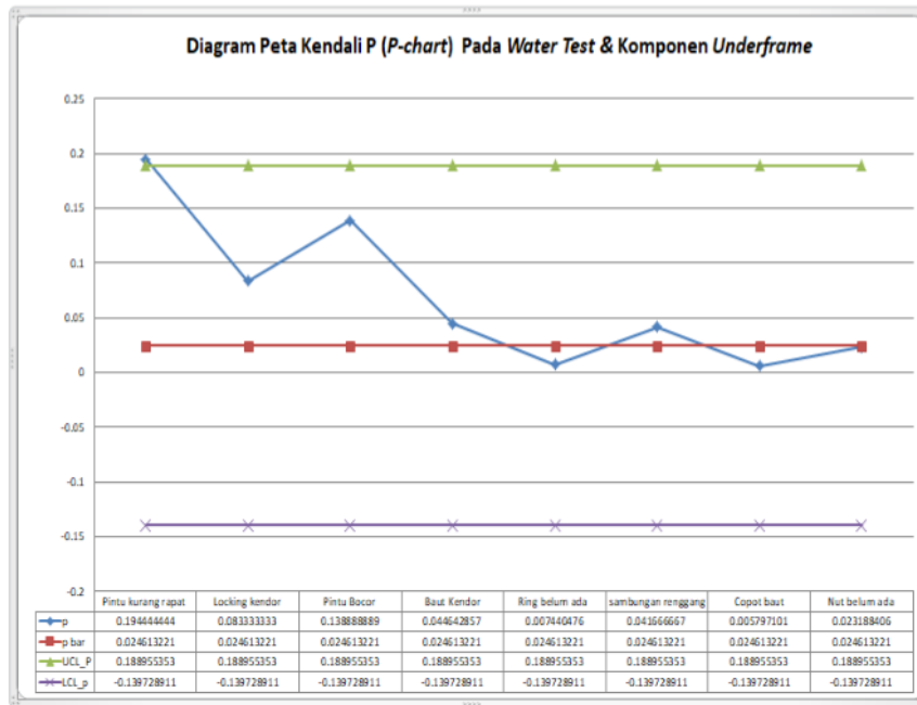
Gambar 2. Peta Kendali Peta Kendali Pada Water Test & Underframe (Sumber: Data Olahan, 2019)
