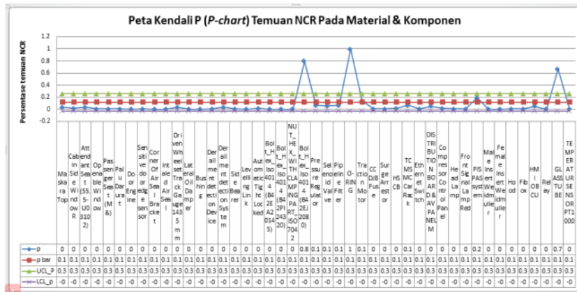
Gambar 4. Peta Kendali Temuan NCR (Sumber: Data Olahan, 2019)
