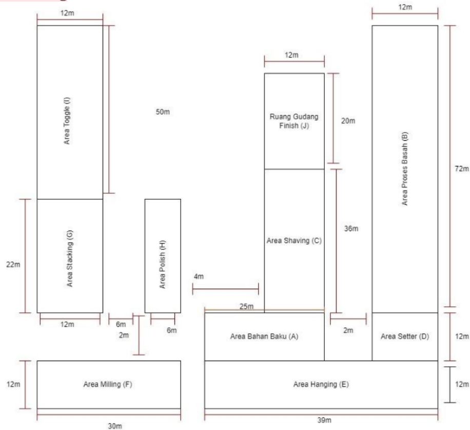
Gambar 2 Layout Sekarang PT Adi Satria Abadi
