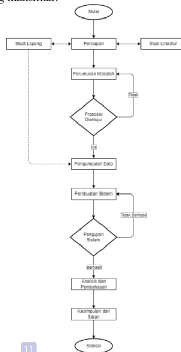
Gambar 1. Tahapan penelitian
