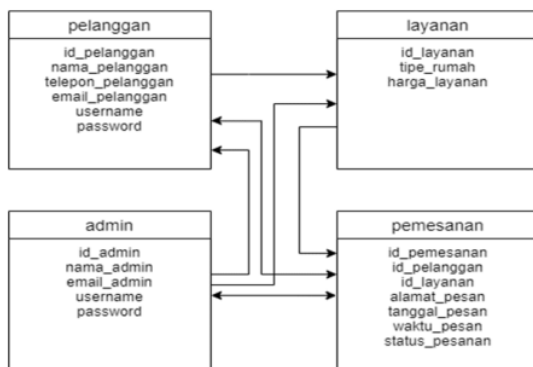
Gambar 6. Relasi Tabel
