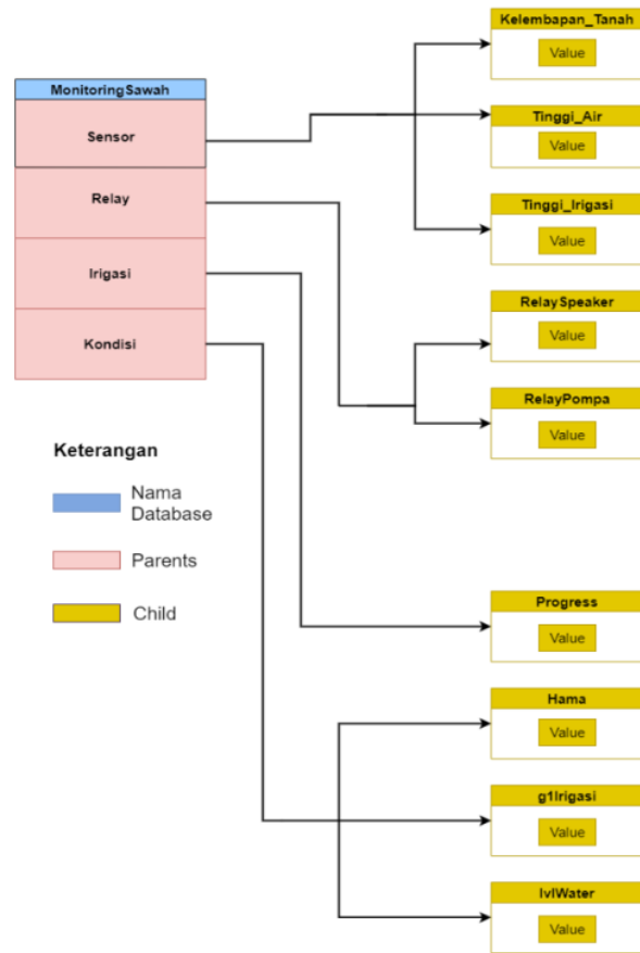
Gambar 6. Model database hirarki pemantauan sawah
