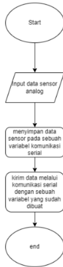
Gambar 7. Flowchart Arduino Uno R3
