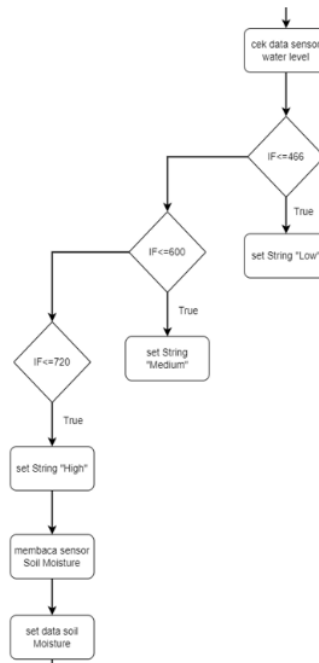
Gambar 8 (b). Flowchart ESP8266 (lanjutan)
