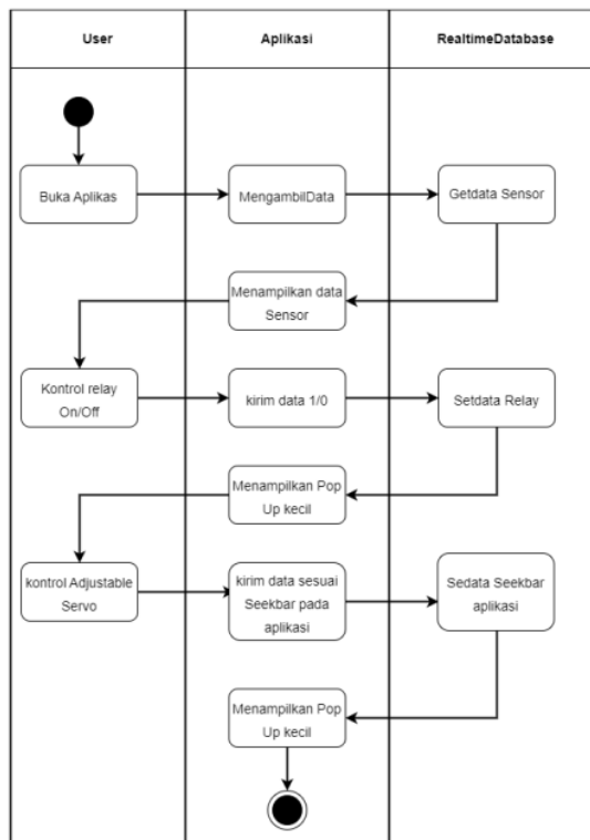
Gambar 4. Activity Diagram Penggunaan Aplikasi
