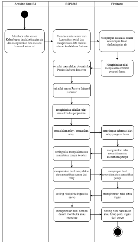
Gambar 5. Activity Diagram komunikasi antara Arduino,ESP8266 dan Firebase
