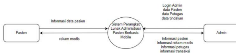
Gambar 4. Diagram Konteks
