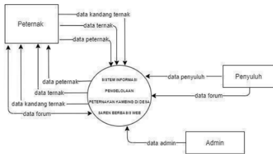
Gambar 1 Diagram Konteks
