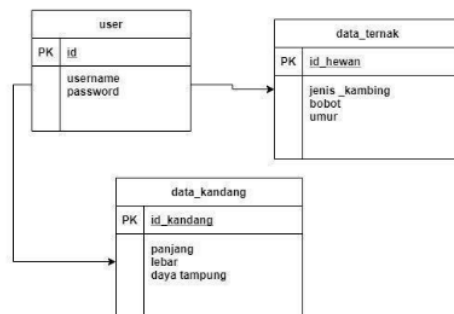
Gambar 2 ERD
