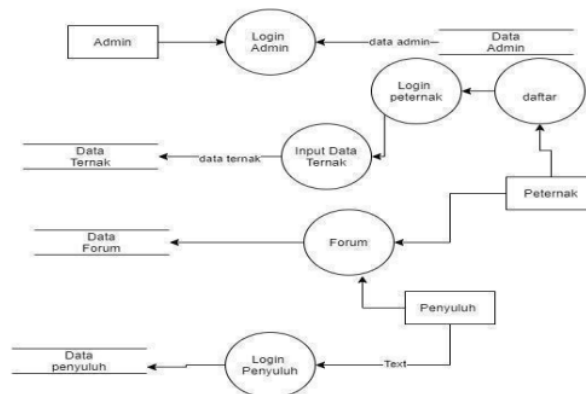
Gambar 3 DFD
