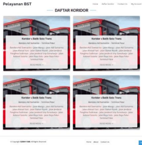
Gambar 5. Daftar Koridor
