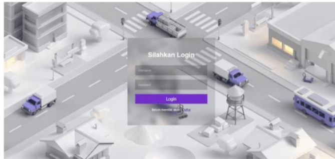
Gambar 3. Halaman Login
