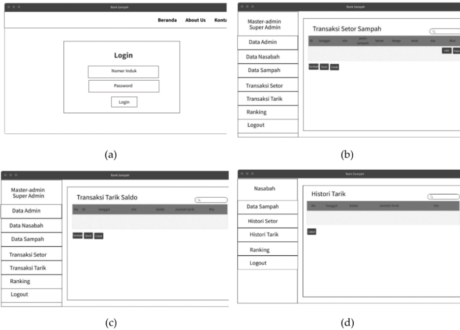
Gambar 4. Rancangan Desain Antarmuka Sistem Informasi Bank Sampah
