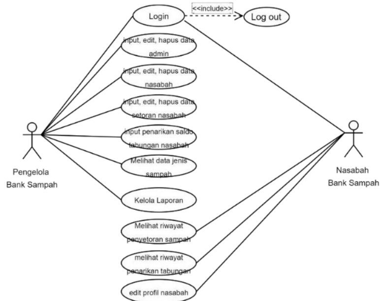
Gambar 2. Usecase Sistem Informasi Bank Sampah
