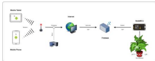
Gambar 1. Arsitektur IoT Aplikasi Monitoring
