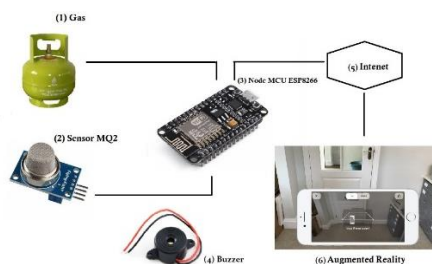
Gambar.3 Rancangan hardware dan software
